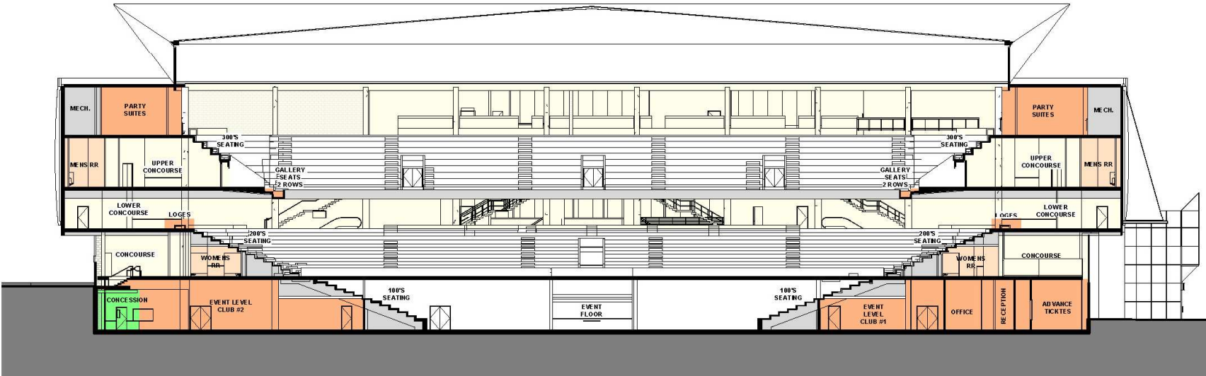
2 Cross Section 1 : 420
